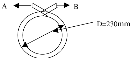
图 1 取样软管较缠试验示意图
